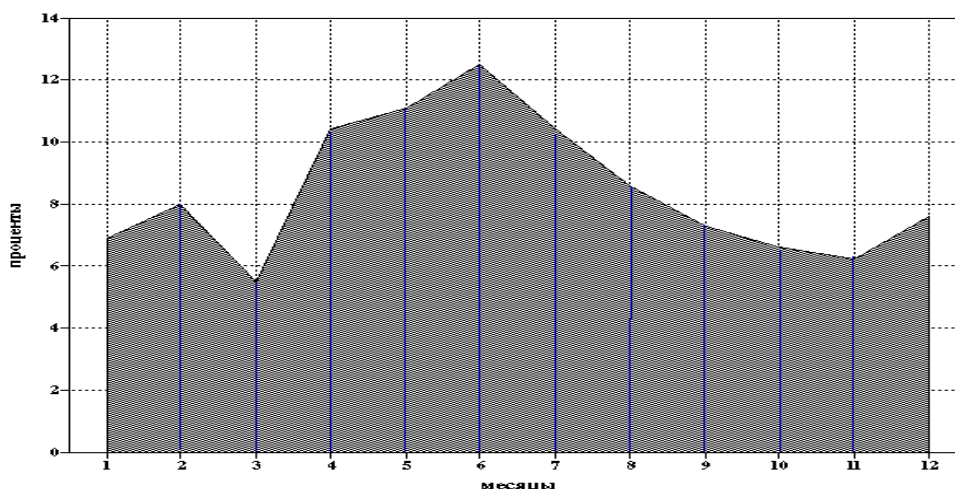
Рис.2-1. Распределение числа извержений вулканов по месяцам года (N=10000).
