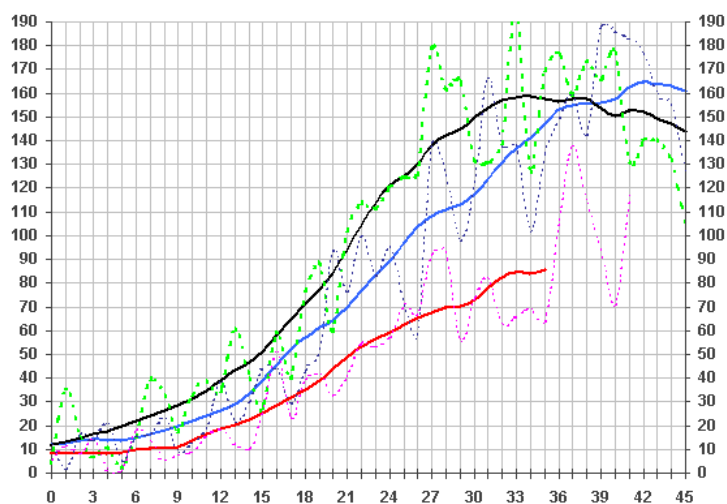
Рис.1. Выход на максимум солнечной активности 21, 22 и 23-го Солнечного циклов.
